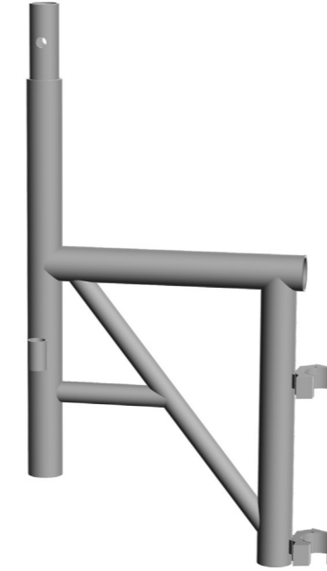
0,30 m H Tipi İskele Kelepçeli Çalışma Konsolu 0,30 m Scaffold Bracket ( With Clamp)
