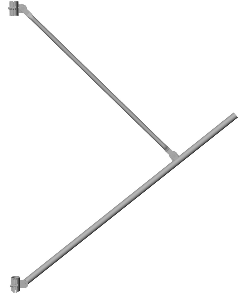
H İskele Taş Koruma Konsol Elemanı Fall Protection Console For H Frame
