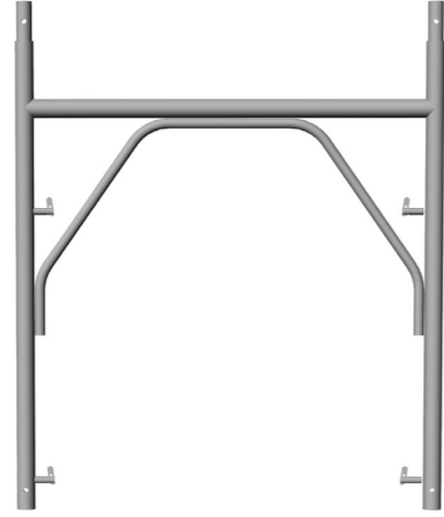
2,00 m H Dar Başlangıç Çerçeve Konsolu 2,00 m Upper Narrow Starting Frame
